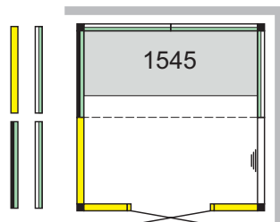
Panacea 1717 dim. : 1700 x 1700 mm
