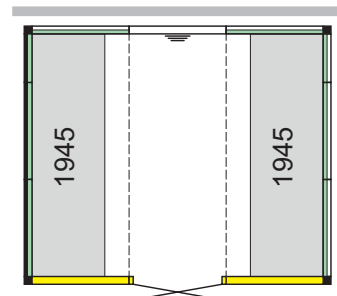
Panacea 2521-2B dim. : 2500 x 2100 mm
