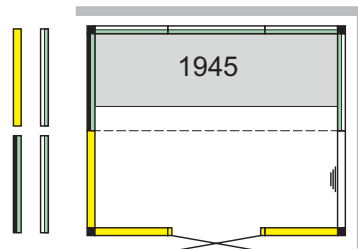
Panacea 2117-1B dim. : 2100 x 1700 mm
